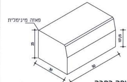
אבן שפה רחבה 50/30/25 * ניתן לקבל מסותת ** ניתן לקבל בשיפוע מותאם לגובה מדרכה 10ס"מ / + 15ס"מ
