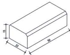
אבן מעבר חציה 23/50/15 * ניתן לקבל מסותת ** ניתן לקבל ללא פאזה
