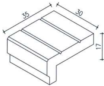
מדרגה מחורצת 17/35/30
