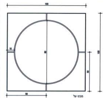
גומה לעץ 100/100 קוטר 80
