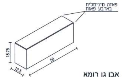
אבן גן רומא 12.5/50/18.75 * ניתן לקבל מסותת
