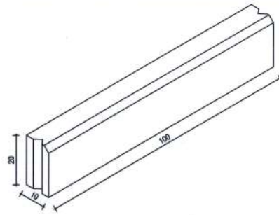
אבן גן 10/20/100 * ניתן לקבל מסותת ** ניתן לקבל ללא פאזה
