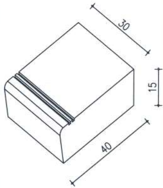
מדרגה נגישה 30/40/15
